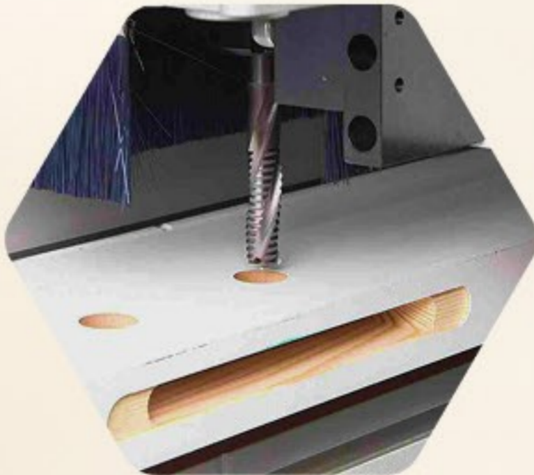
Door CNC
